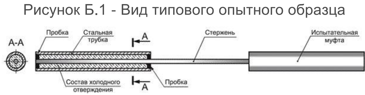
Рисунок Б.1 - Вид типового опытного образца
