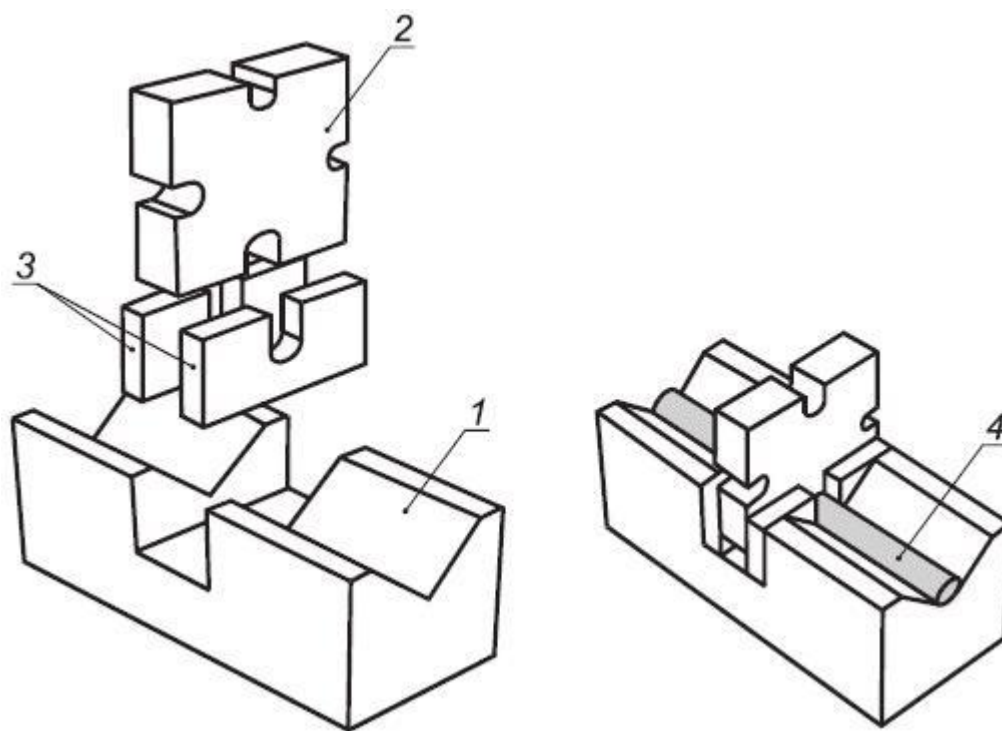
Рисунок Г.1 - Приспособление для испытания образцов на поперечный срез
